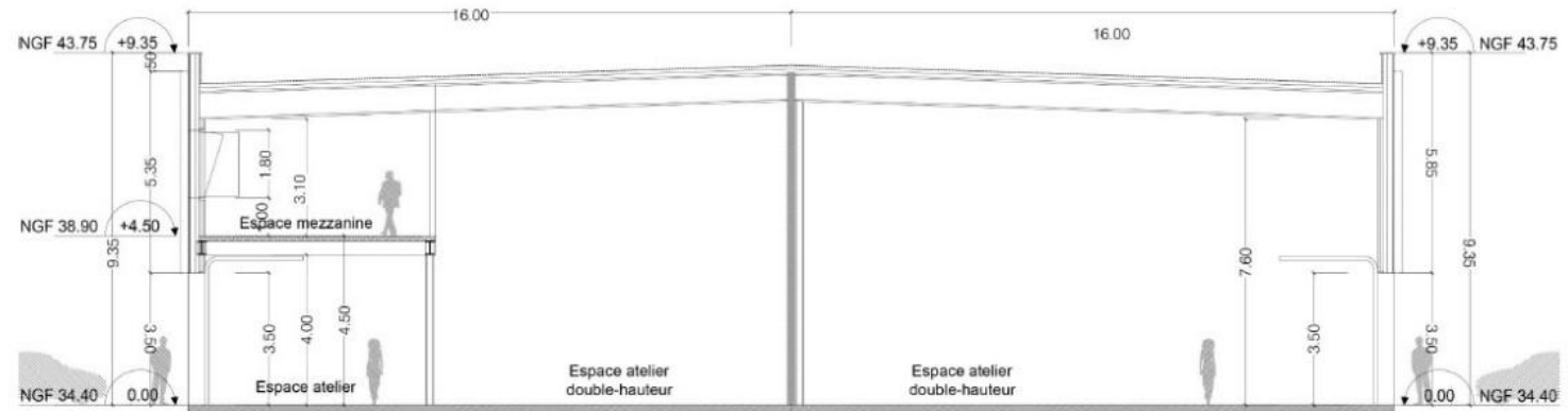
COUPE TRANSVERSALE BAT A - ATELIERS
