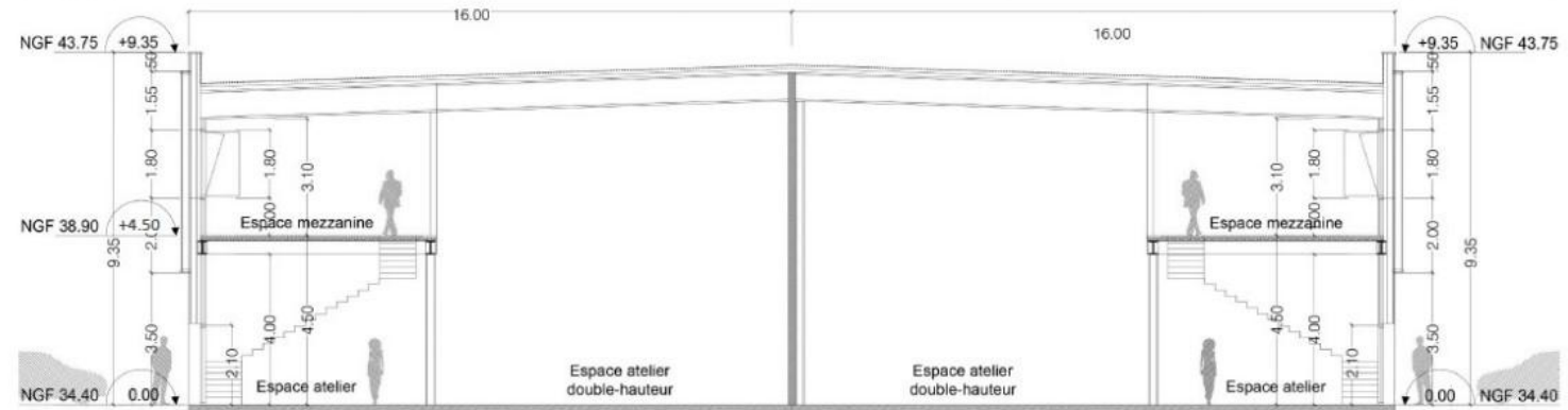
COUPE TRANSVERSALE BAT A - MEZZANINES
