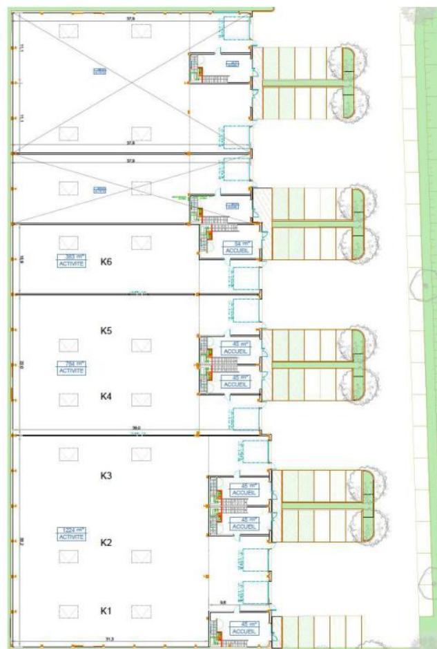
PLAN RDC
